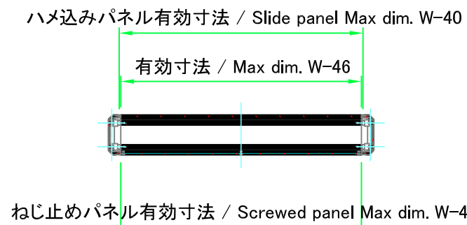
A-A (1 : 10)
