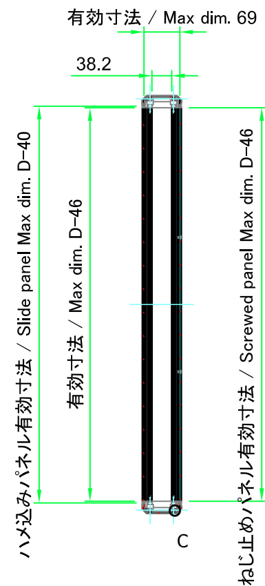
B-B (1 : 10)
